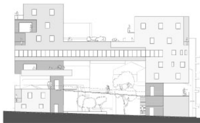
Τίνα Δογάνη / Πολυκατοικία Tina Dogani / Polykatoikia καθ. Δ. Κατούτα - prof. D. Katsota / 2011
