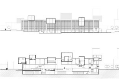
Θεοδώρα Παπαμιχαήλ / Βιβλιοθήκη Πολυμέσων Theodora Papamichail / Mediateque καθ. Π. Δραγώνας - prof. P. Dragonas / 2010
