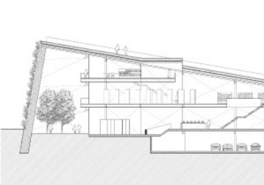
Εμίλη Κουσταή / Βιβλιοθήκη Emily Koustae / Library καθ. Δ. Γιαννιάς - prof. D. Giannisis / 2010
