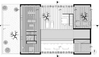
Κάλλια Φυσάρη / Κατοικία με χώρο εργασίας Kallia Fysaraki / Single-family House with Working Space καθ. Σ. Γιαννίκης - prof. S. Giannikis / 2009
