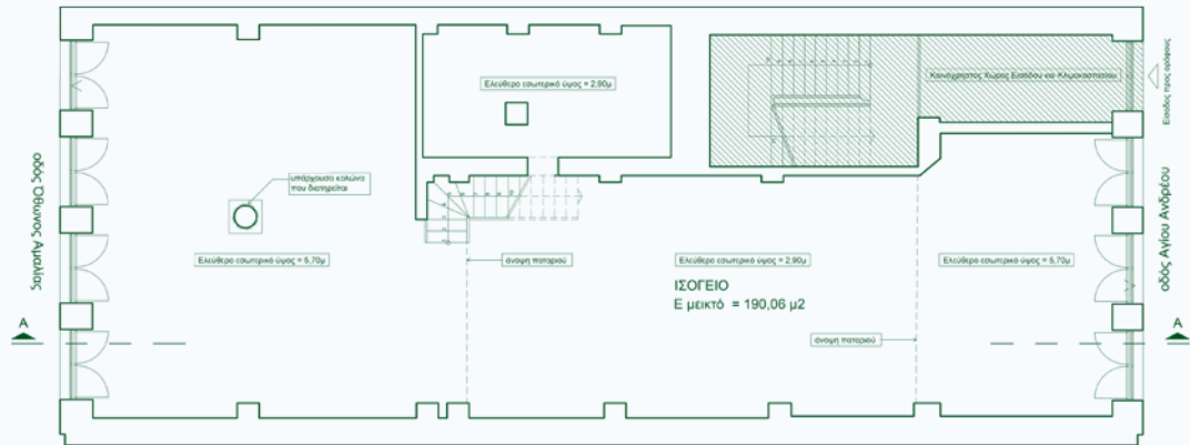
ΧΩΡΟΣ Α, ΥΠΑΡΧΟΥΣΑ ΚΑΤΑΣΤΑΣΗ, ΚΑΤΟΨΗ ΙΣΟΓΕΙΟΥ
