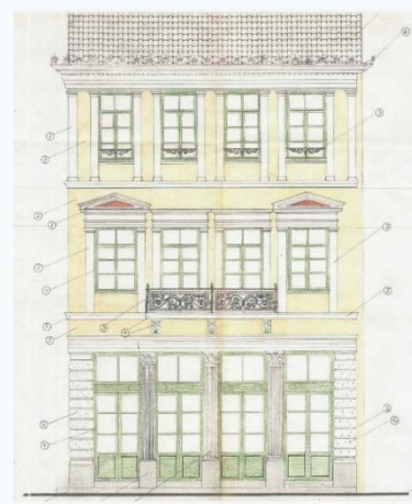
Εικόνα 4: Σχέδιο Όψης επί της οδού Όθωνος Αμαλίας (1996)
