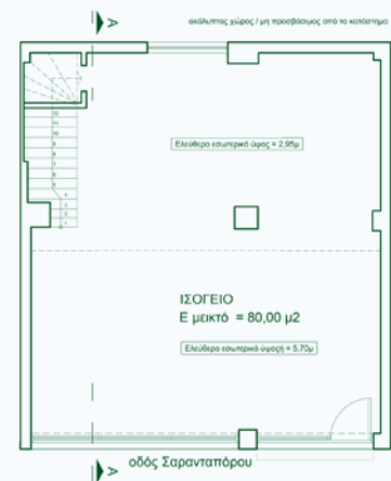
ΧΩΡΟΣ Β, ΥΠΑΡΧΟΥΣΑ ΚΑΤΑΣΤΑΣΗ, ΚΑΤΟΨΗ ΙΣΟΓΕΙΟΥ
