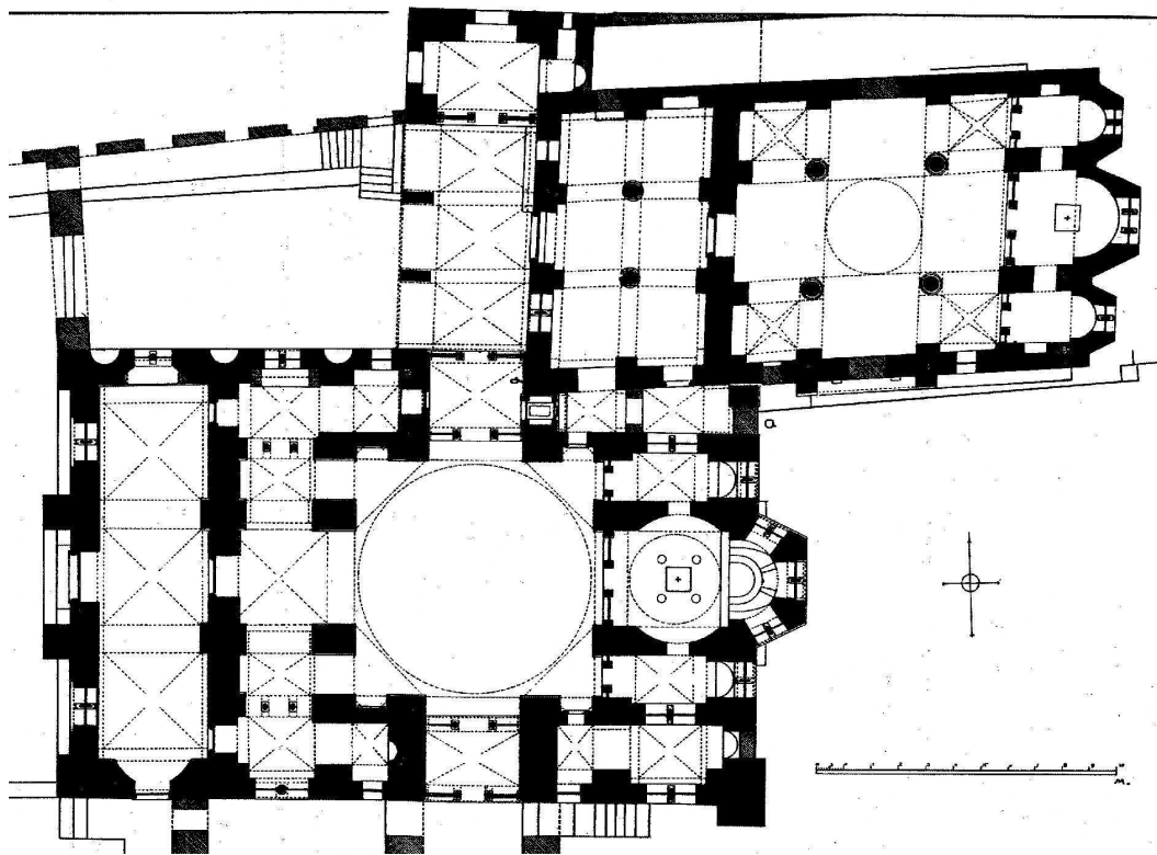
Μονή Οσίου Λουκά. Καθολικό & Ναός Παναγίας. Κάτοψη (Schultz - Barnsley).
