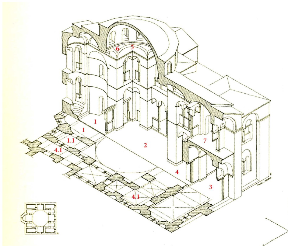
Μονή Οσίου Λουκά. Καθολικό. Αξονομετρική τομή (Κουφόπουλος - Μυριανθέως).
