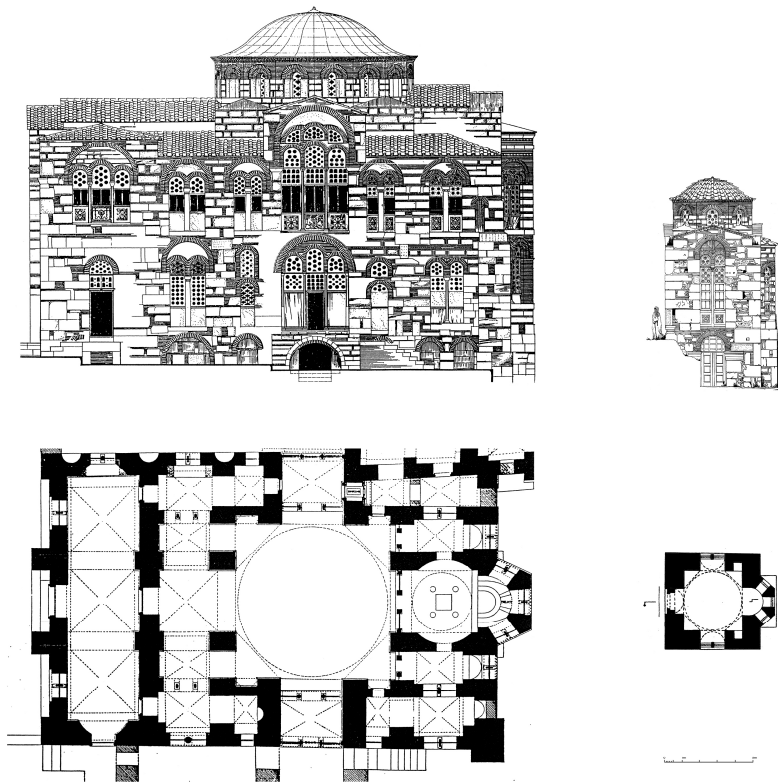
Μονή Οσίου Λουκά. Καθολικό & Ναΐσκος. Κάτοψη & Ν. Όψη (Schultz - Barnsley).
