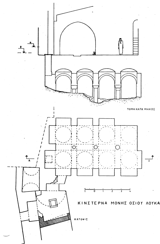
Μονή Οσίου Λουκά. Δεξαμενή. 11 ος αι. (Μπούρας).
