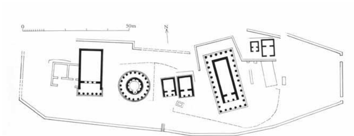
Δελφοί. Ιερό Προναίας Αθηνάς. Τοπογραφικό.
